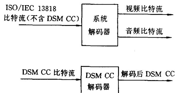
图 I-A-2 DSM CC 做为单独比特流被解码
