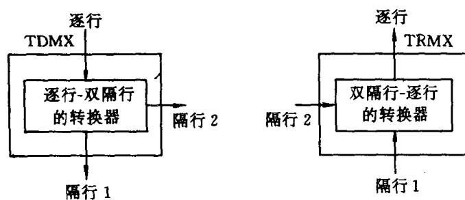
图 I-D-5 对于“逐行；隔行-隔行时域分级”的时域分解器和再复合器
