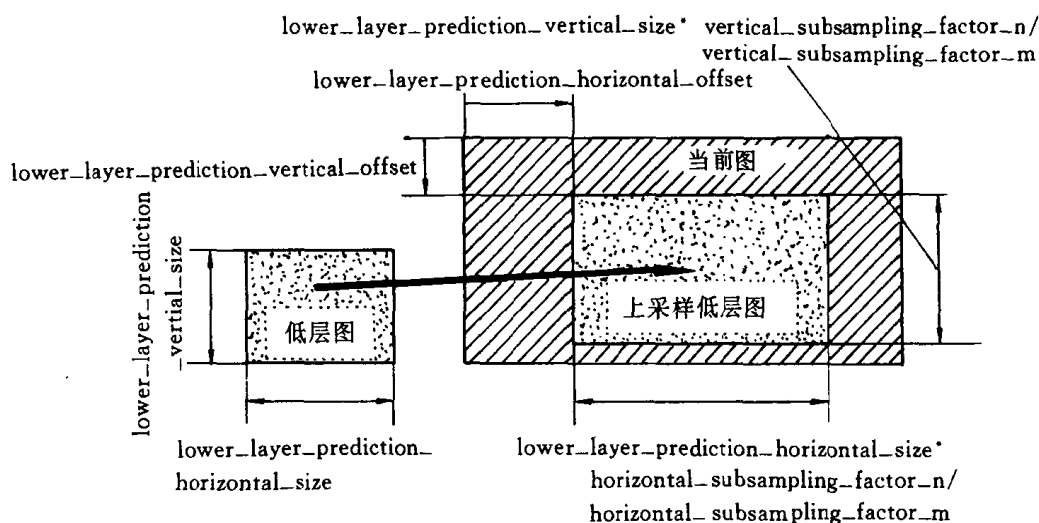
图 Ⅱ-7-14 通过对低层图插值得到的“空域”预测结构
