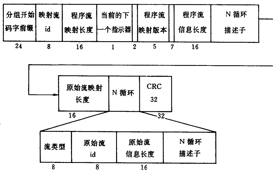
图 I-F-8 程序流映射图
