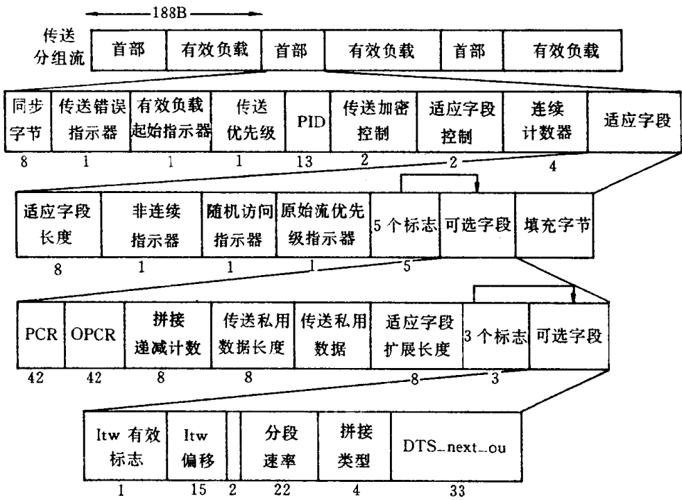
图 I-F-1 传送流语法图
