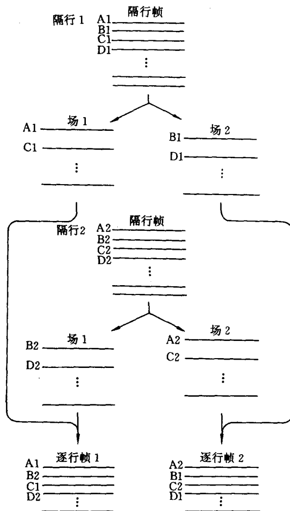
图 I-D-4 双隔行—逐行的转换
