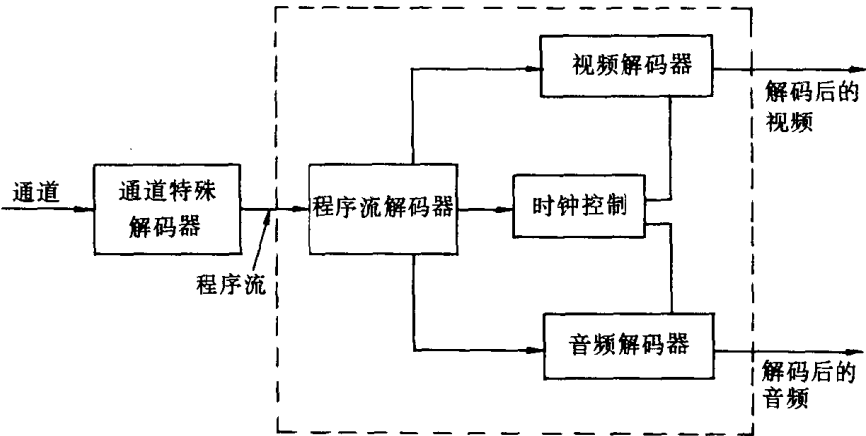
图 I-0-5 程序流原型解码器
