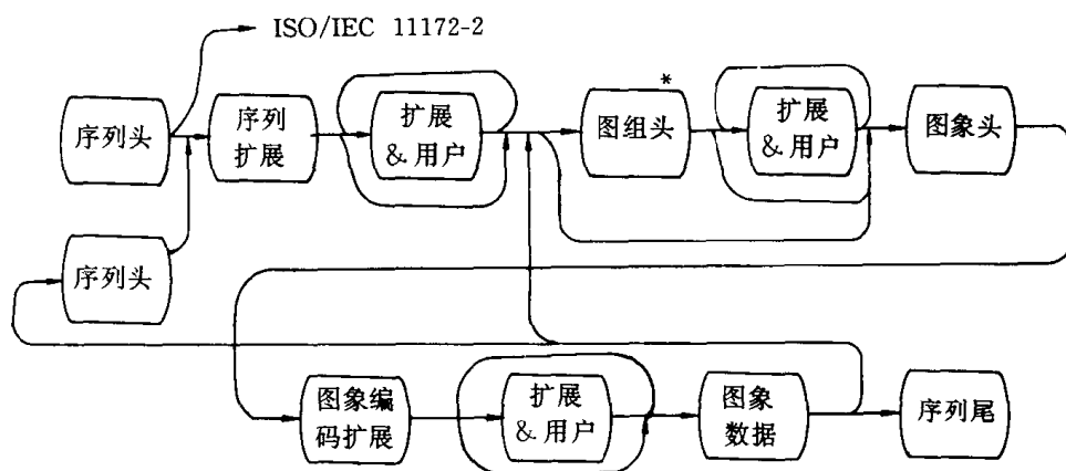
图 I-6-15 高层比特流组织
