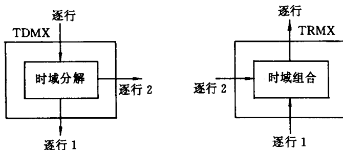
图 I-D-2 对于“逐行：逐行-逐行时域分级”的时域分解器和再复合器
