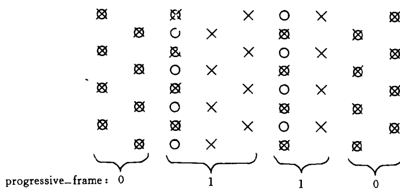
图 I -7-22 色差格式为 4:2:2 或 4:4:4, progressive_sequence==0
