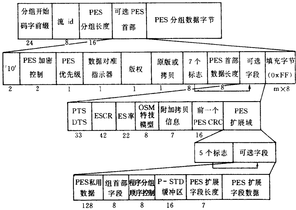
图 I-F-2 PES 分组语法图
