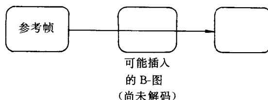
图 II -7-10 I-图和 P-图的帧预测
