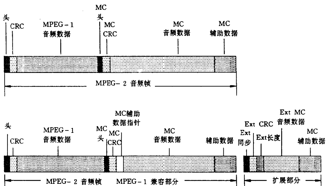
图 III-A-2 ISO 13818-3 多通道扩展层 II 结构,使用 ISO/IEC 11172-3 兼容比特流和扩展比特流
