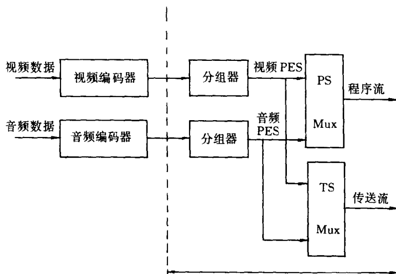
图 I-0-1 ITU-T Rec. H. 222.0|ISO/IEC 13818-1 简化的总体框图
