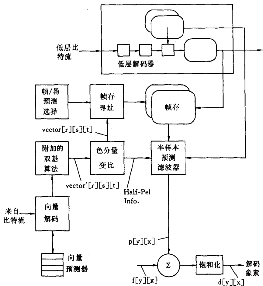
图 I -7-16 使用时分域分级的对增强层的运动补偿过程的简化图
