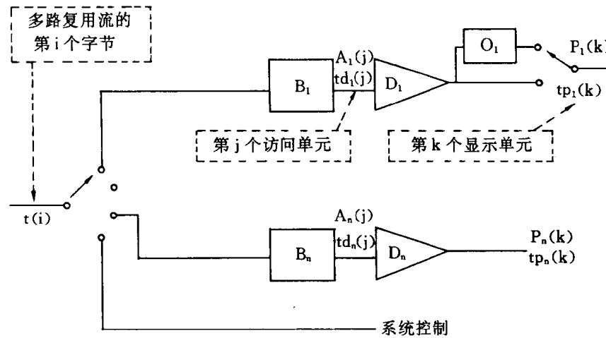
图 1-2-7 程序流系统目标解码器的表示法
