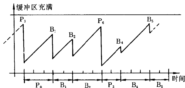
图 II-C-2 只有 P,B 图时 VBV 的一种简单情况
