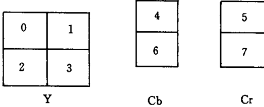
图 I-6-11 4:2:2 宏块结构
