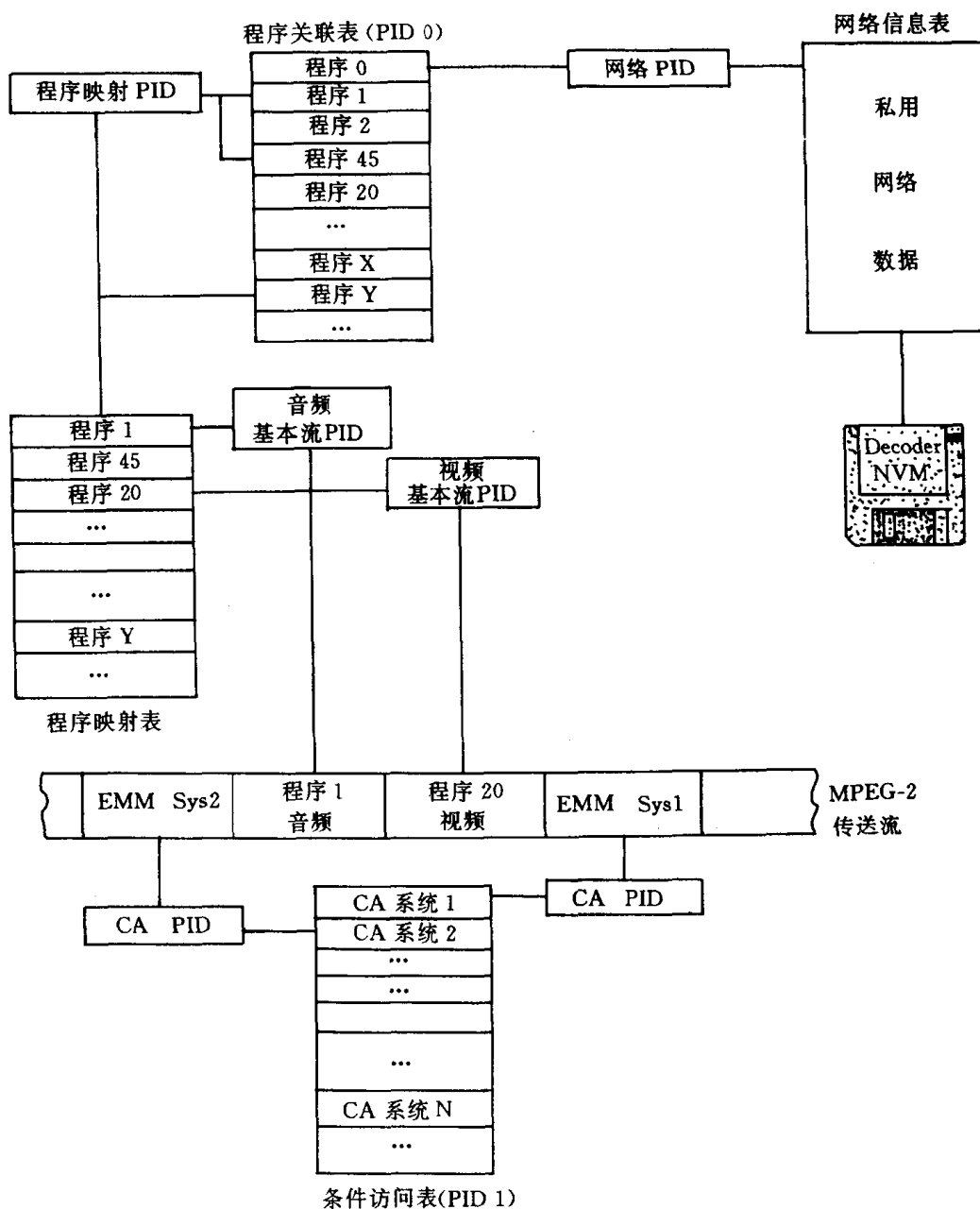
图 I-C-1 程序和网络映射关系
