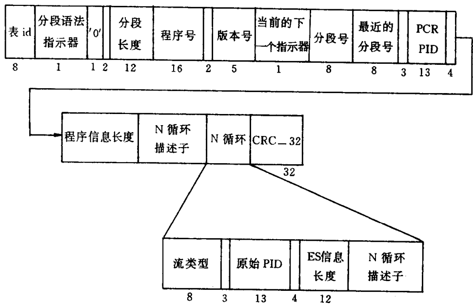
图 I-F-5 TS 程序映射图
