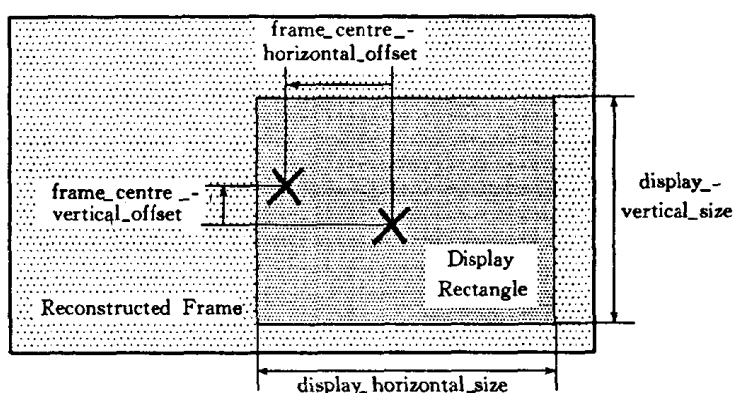
图 II-6-16 帧中心偏移参数
