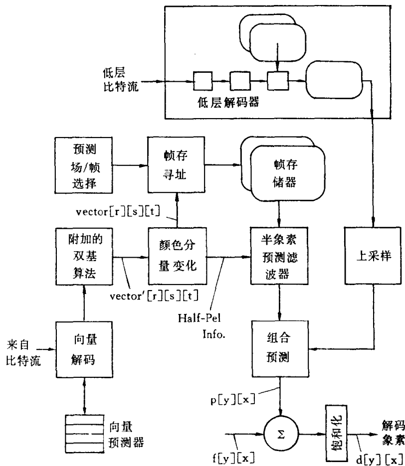
图 II-7-13 空域分级的简化的运动补偿过程
