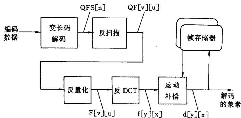
图 II-7-1 简化的视频解码过程
