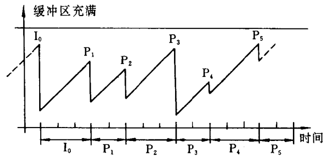
图 II -C-3 只有 I,P 图时 VBV 的一种简单情况
