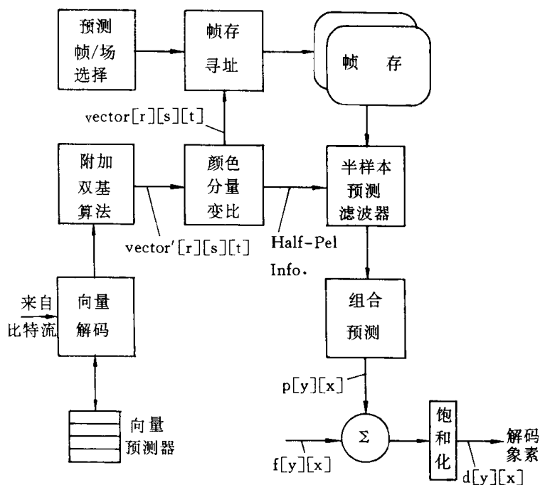
图 II-7-5 简化的运动补偿过程
