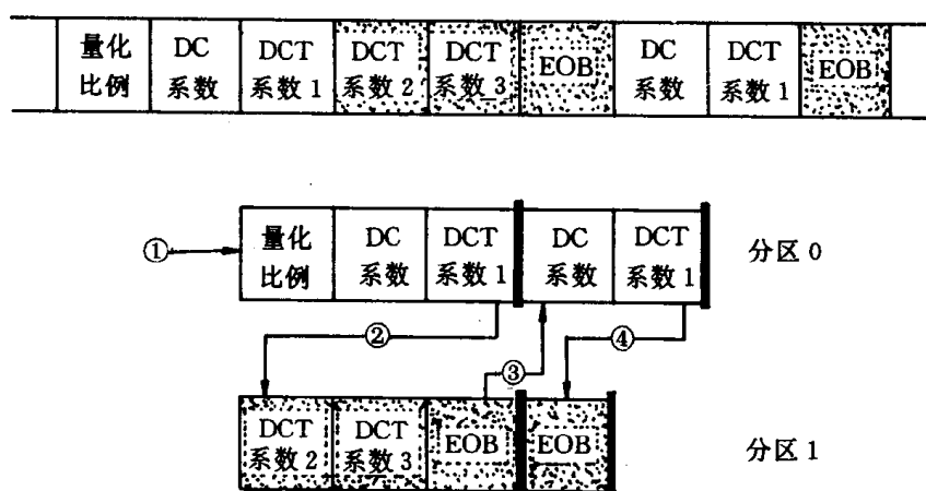
图 II-7-17 priority_breakpoint 置为 64(一对(run,level)), 带有两个分区的比特流的分割。两个分区如图所示, 用箭头指出解码器需要如何在两分区间切换
