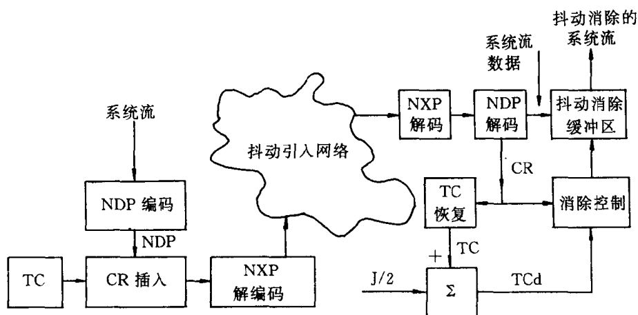
图 I-K-2 使用网络层时间标签进行抖动平滑
