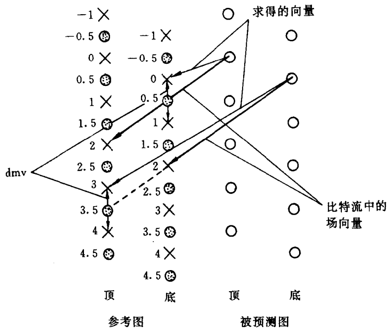
图 I -7-12 双基预测的运动向量变化
