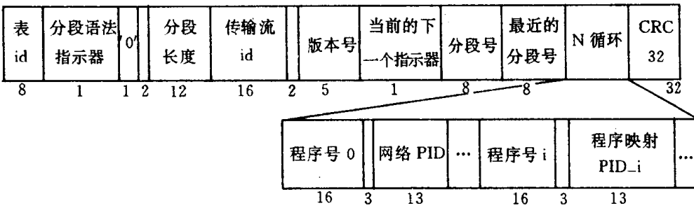
图 I-F-3 程序关联分段图
