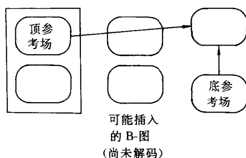
图 II-7-8 当第二个场图为顶场时的预测
