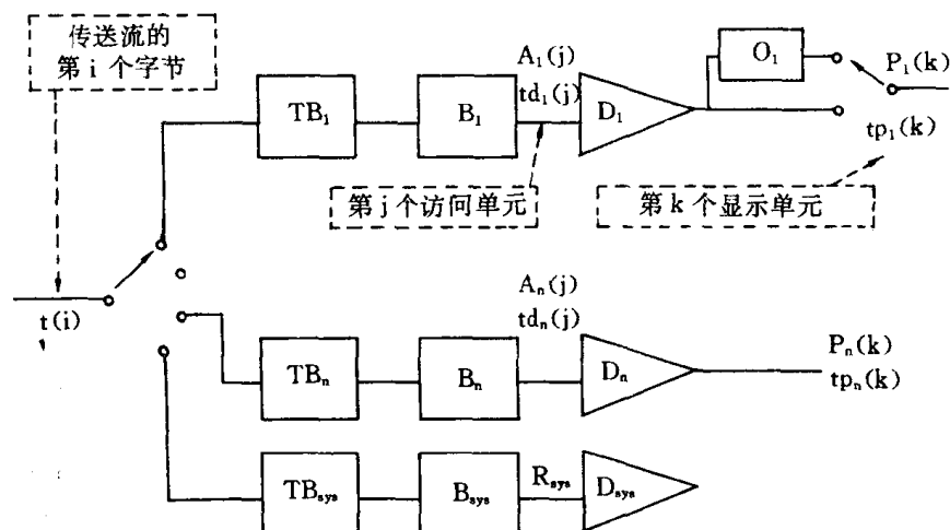
图 1-2-6 传送流系统目标解码器的表示法
