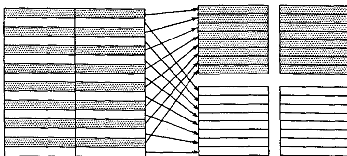
图 I-6-14 在场 DCT 编码中的亮度宏块结构
