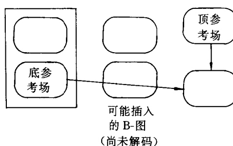
图 II-7-7 当第二个场图为底场时的预测
