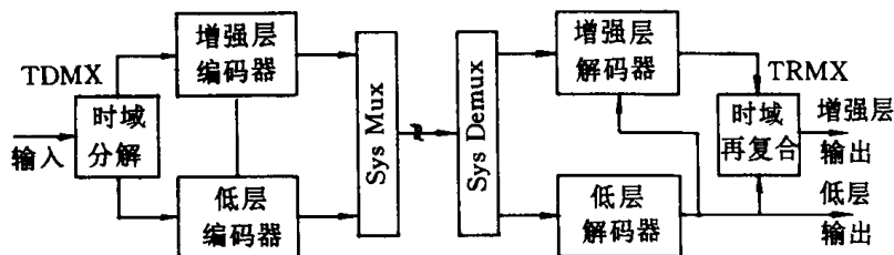
图 I-D-1 针对时域分级的双层编码解码结构
