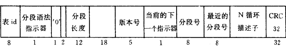
图 I-F-4 条件访问分段图
