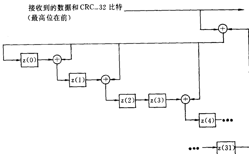
图 I-B-1 32 比特 CRC 解码器模型
