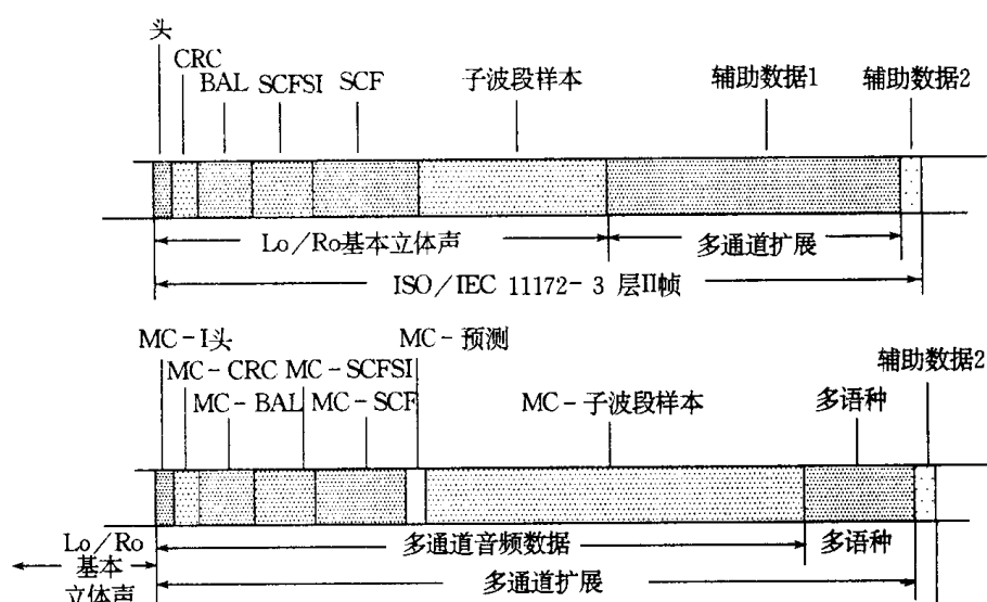
图 III-A-1 ISO 13818-3 层 II 多通道扩展结构,与 ISO 11172-3 层 II 向后兼容
