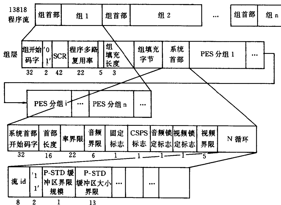
图 I-F-7 程序流图
