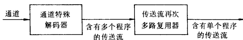
图 I-0-3 典型的传送多路复用示例
