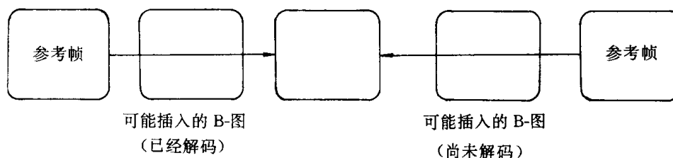
图 II -7-11 B-图的帧预测
