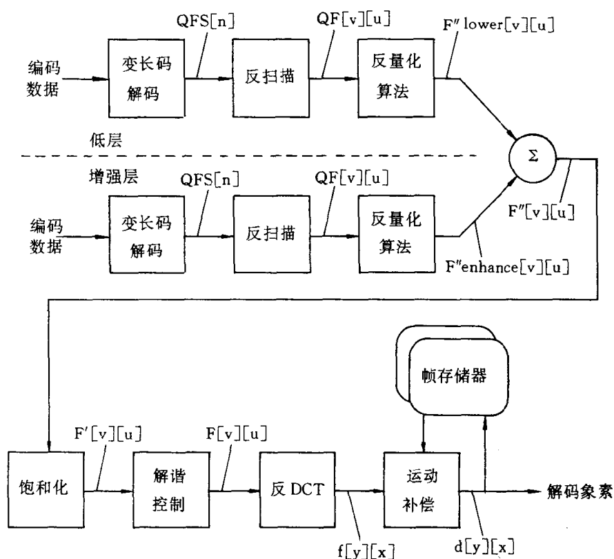
图 II-7-15 SNR 分级解码过程描述
