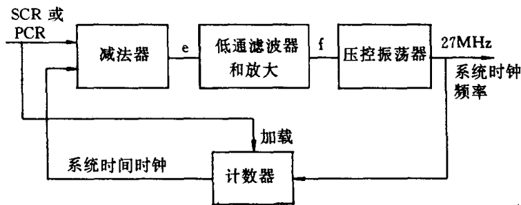
图 I-D-2 使用 PLL 的 STC 恢复
