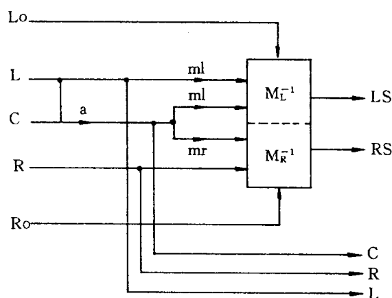
图 III-1 联合立体声逆矩阵的修改过程
