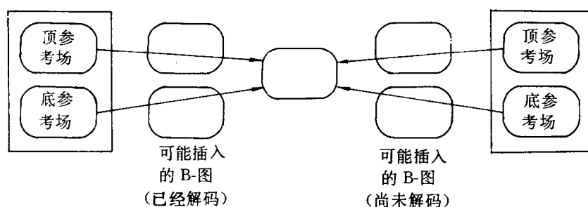
图 II -7-9 B 帧图或 B 场图的场预测
