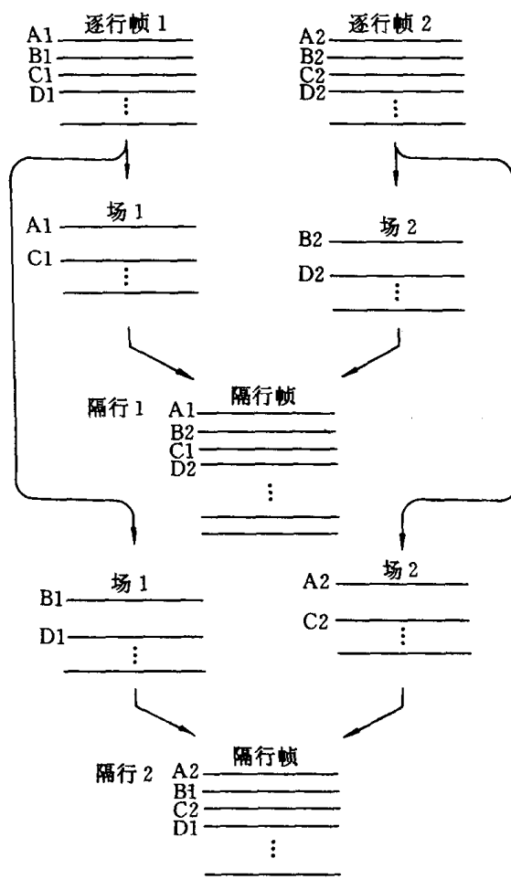
图 I-D-3 逐行—双隔行的转化
