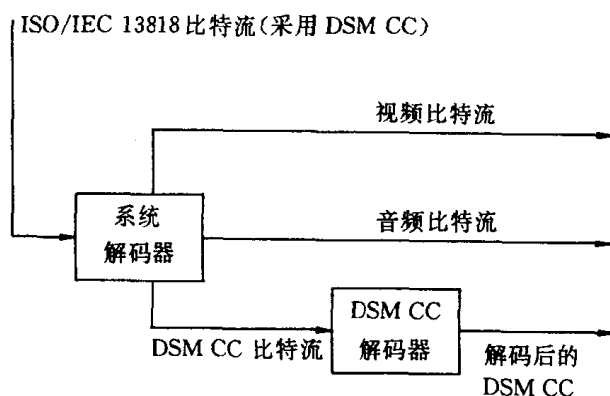
图 I-A-3 DSM CC 做为系统比特流的一部分被解码
