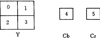
图 I-6-10 4:2:0 宏块结构
