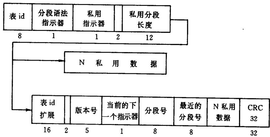
图 I-F-6 私用分段图
