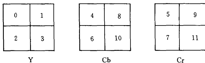
图 I-6-12 4:4:4 宏块结构
