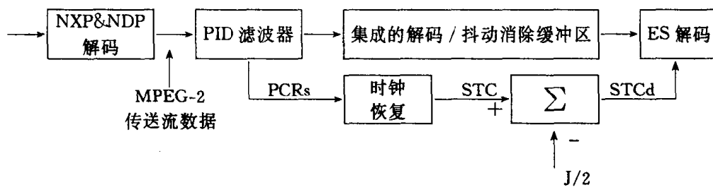
图 1-K-3 集成的抖动消除和 MPEG-2 解码
