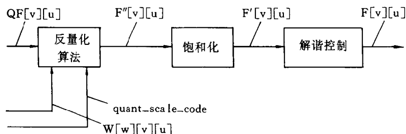
图 II -7-4 反量化过程
