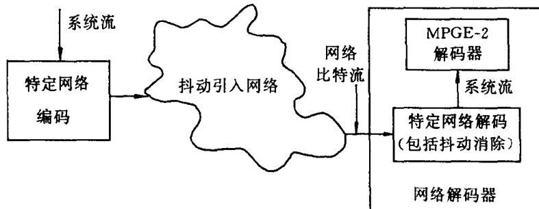
图 I-K-1 在一抖动引入网络中传送系统流
